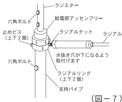
⑨各ラジアルをラジアルリングにネジ込みます。その後、各ラジアルコイルの水抜き穴が下向きになるように戻し、ラジアルナットで固定します。(50MHzのラジアルには水抜き穴がありません)
