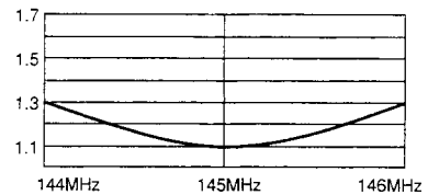
144MHz帯
